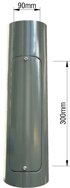
DOOR DETAIL
