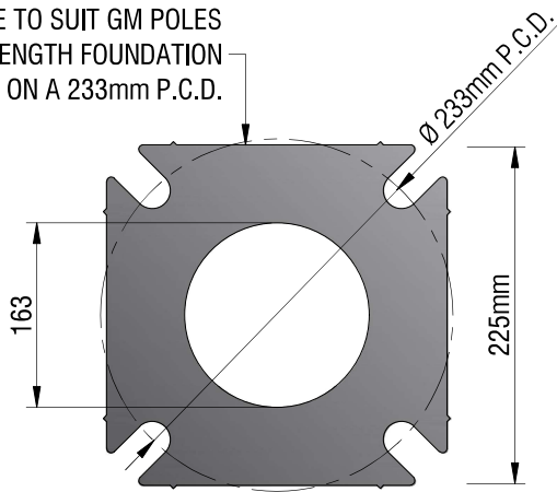
BASEPLATE
