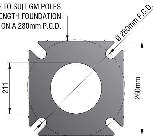
BASEPLATE
