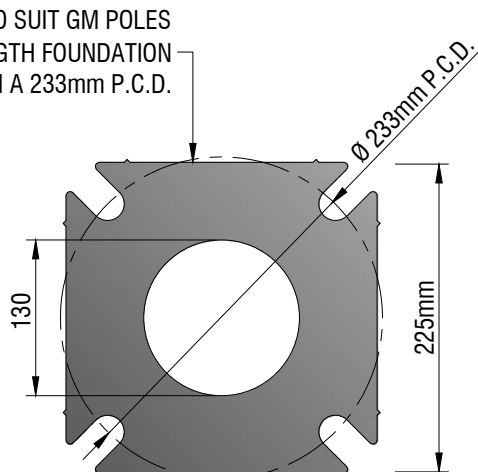
BASEPLATE
