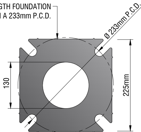
BASEPLATE
