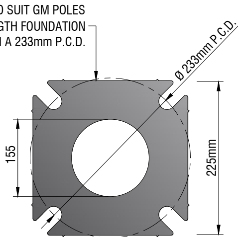
BASEPLATE
