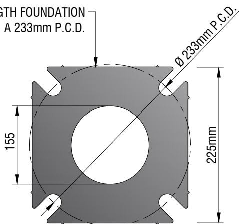
BASEPLATE
